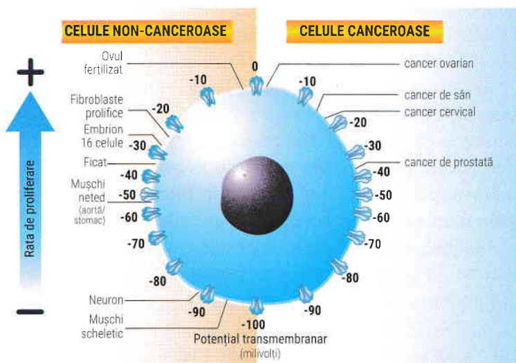
Figura 1. Relația dintre diferența de potențial electric a celulelor de-a lungul membranei lor și capacitatea de a se înmulți rapid. Celulele din medii cu creștere rapidă (de exemplu, embrionii) se caracterizează prin diferențe de potențial cu valori negative mici, în timp ce au valori negative mai mari celulele mai mature. Nu este surprinzător că toate celulele tumorale prezintă valori în intervalul cu valori negative mai mici. 4
